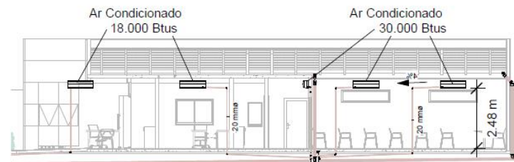
2 Corte 1 1 : 150
