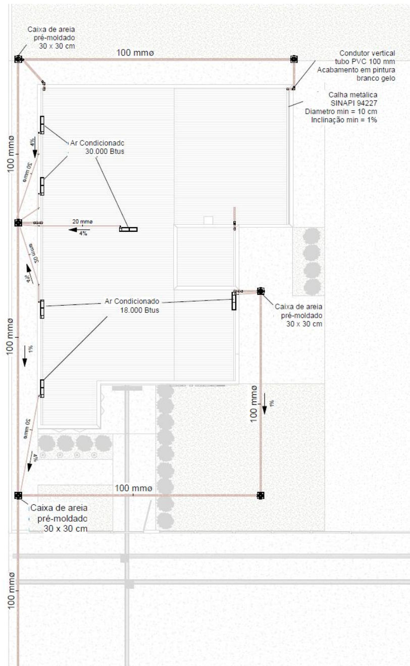
1 Planta de drenagem - Ar 1 : 150
