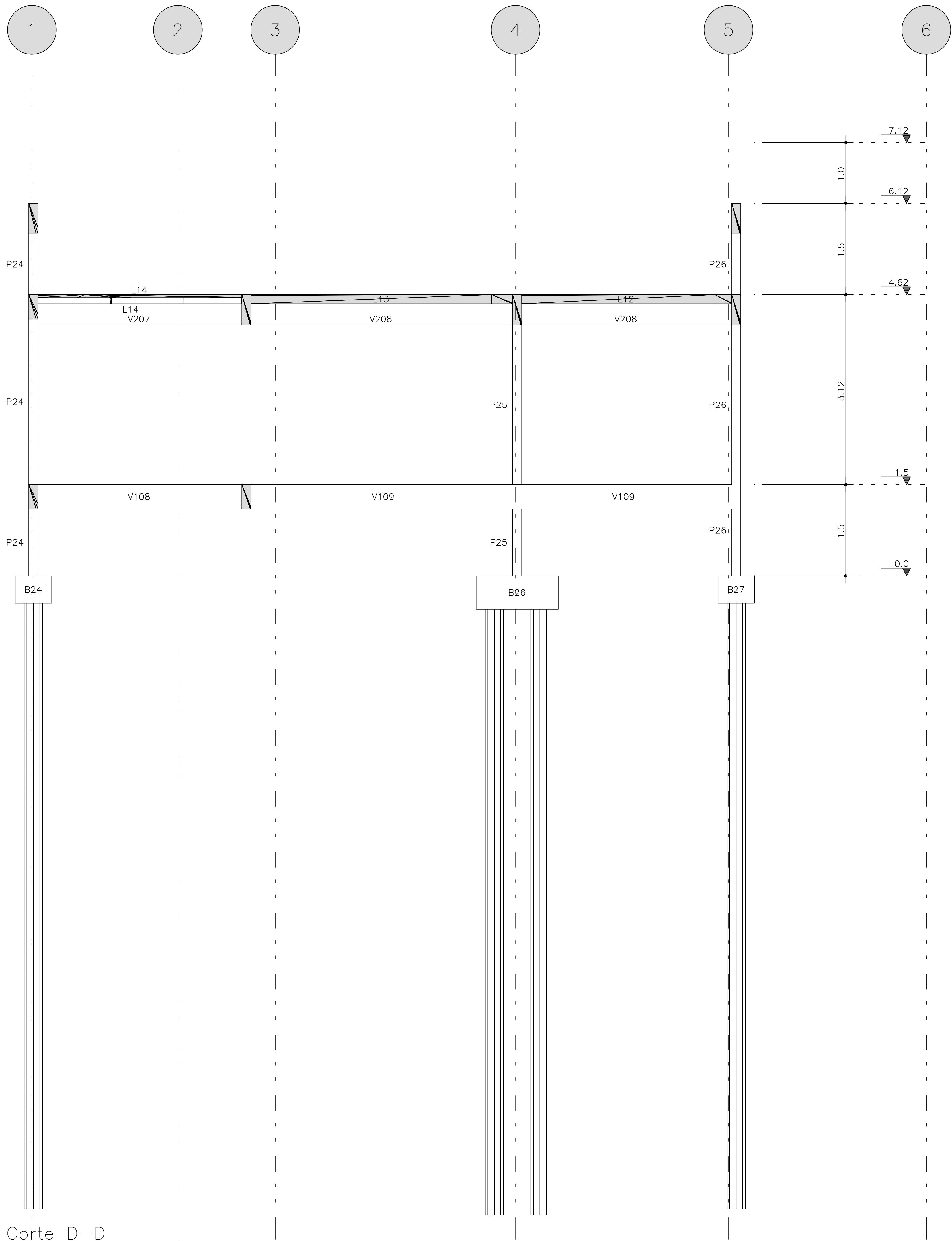
Corte D-D
